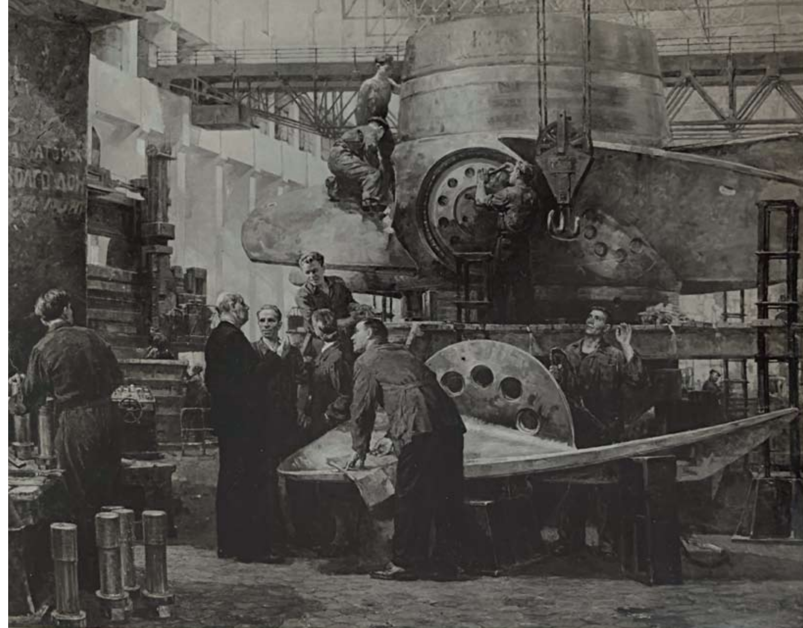
ЛЕНИНГРАД — ВЕЛИКИМ СТРОЙКАМ КОММУНИЗМА. СБОРКА ТУРБИНЫ ДЛЯ ЦИМЛЯНСКОЙ ГЭС НА ЗАВОДЕ ИМ. И.В. СТАЛИНА. 1951 г.
